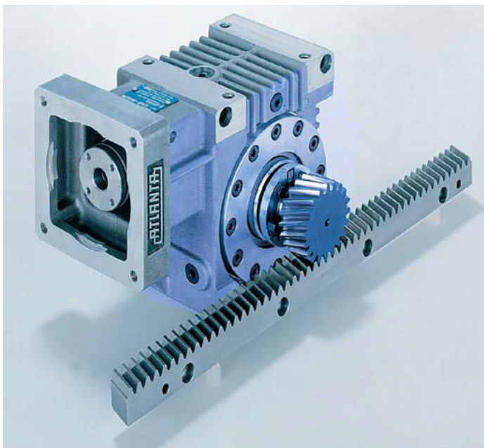
Die Familie der Atlanta-Servoschneckengetriebe ist die breiteste Palette von Servo-Winkelgetrieben mit Hohlwelle, welche derzeit auf dem Markt verfügbar ist. (Bild: Atlanta Antriebssysteme)
