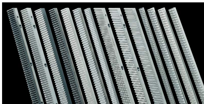
Atlanta verfügt über ein breit gefächertes Zahnstangenprogramm. Rund 300 verschiedene, ab Lager lieferbare Standard-Zahnstangen lassen für den Konstrukteur kaum noch Wünsche offen. (Bild: Atlanta Antriebssysteme)
